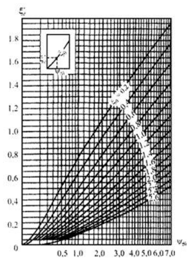
Рисунок K.6 - Графики для определения коэффициента \xi'_e
