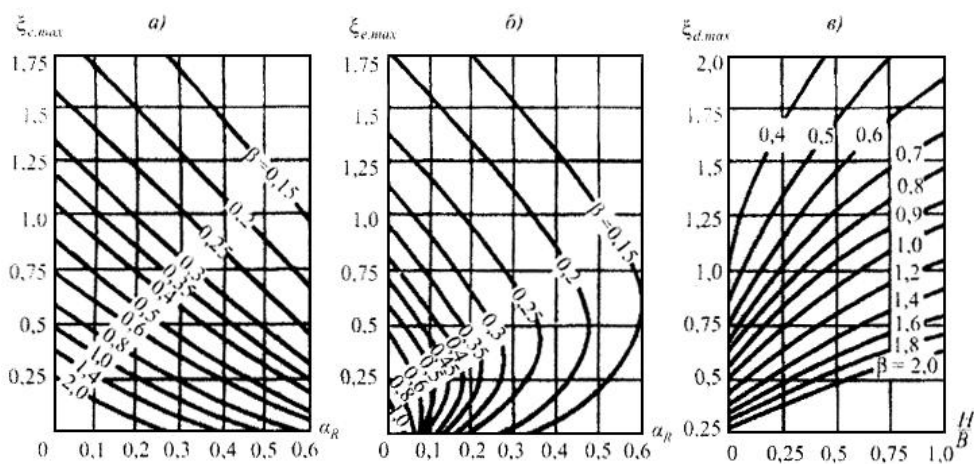
Рисунок К.3 - Графики для определения коэффициентов:
