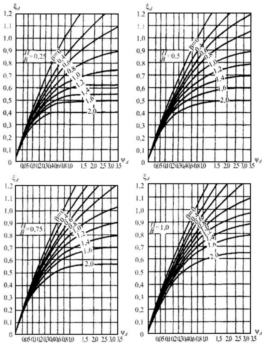
Рисунок К.4 - Графики для определения коэффициента \xi_d
