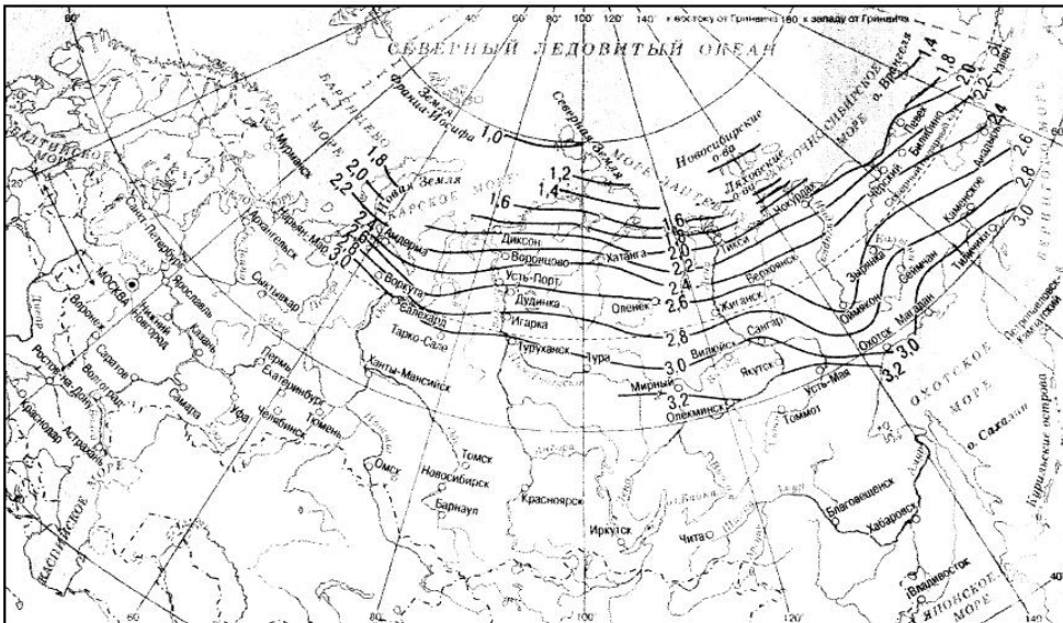
Рисунок Г.1 - Глубины оттаивания песчаных грунтов
