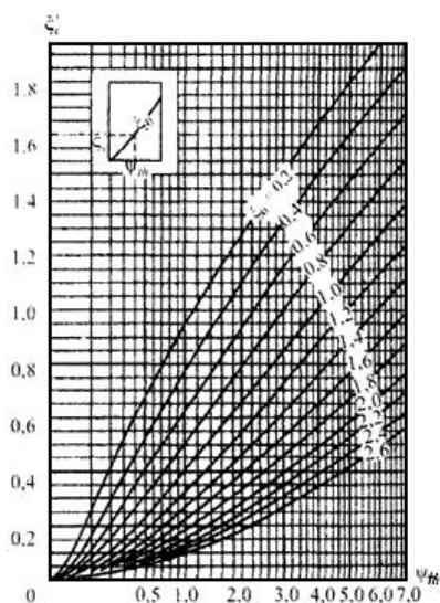
Рисунок K.5 - Графики для определения коэффициента \xi'_c
