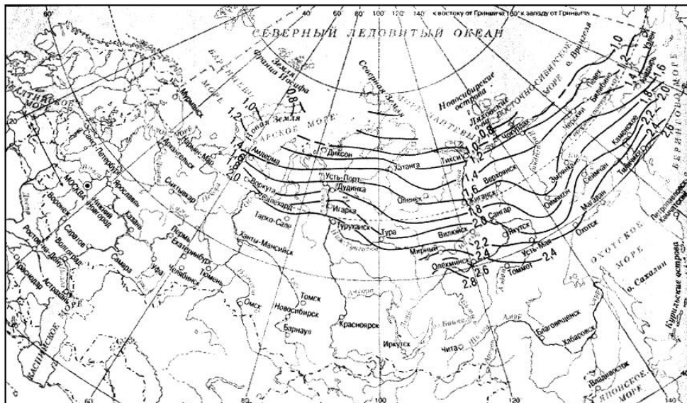
Рисунок Г.2 - Глубины оттаивания глинистых грунтов
