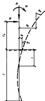
Схема нагрузок на сваю
