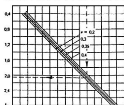
Номограмма для определения значений \delta_0
