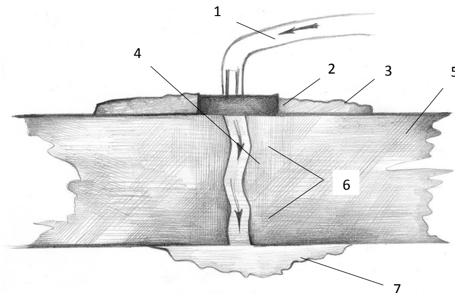
Рисунок 27 – Подача составов в трещину через накладные иньекторы
