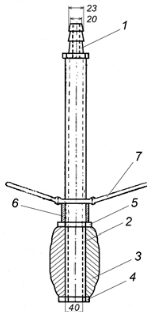
Рисунок 9 – Механический распорный пакер прямой подачи раствора:
