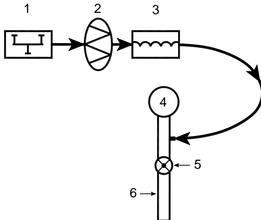
Рисунок 6 – Зажимной способ подачи раствора:
