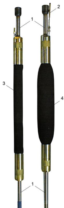
Рисунок 10 – Пакер распорный. Фиксация пакера в отверстии
