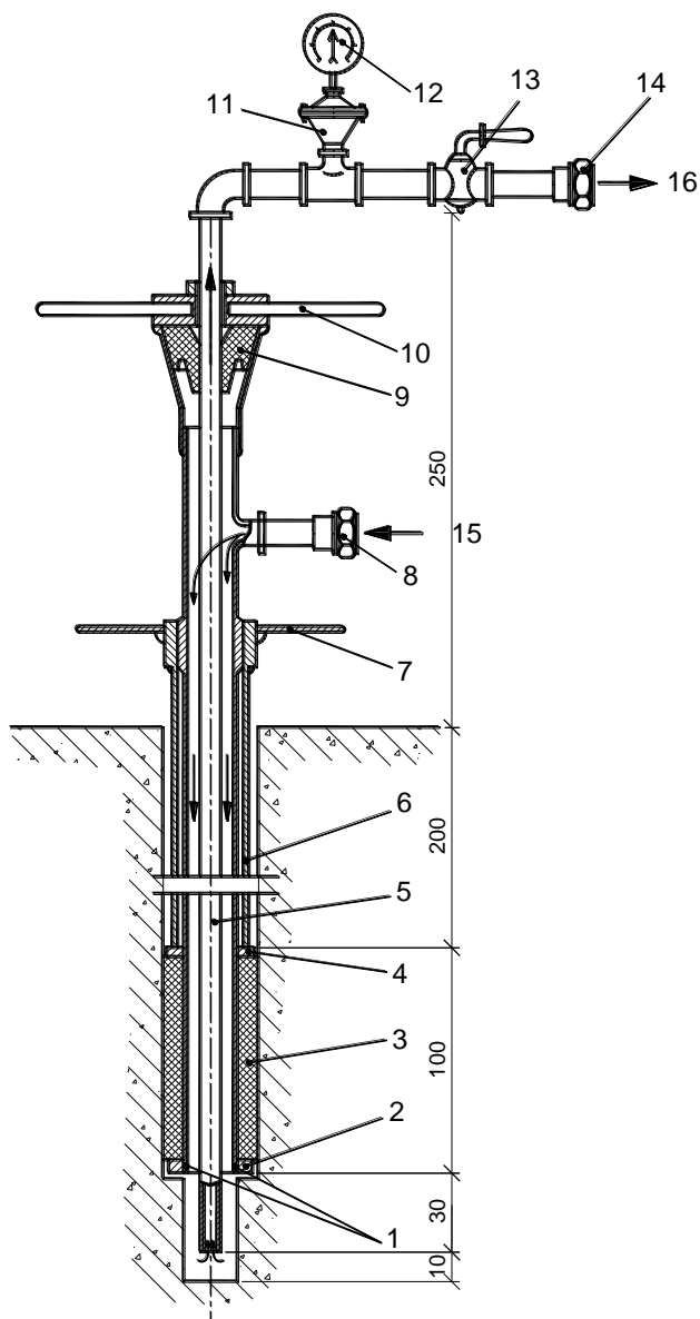
Рисунок 8 – Иньектор с обратной циркуляцией раствора:
