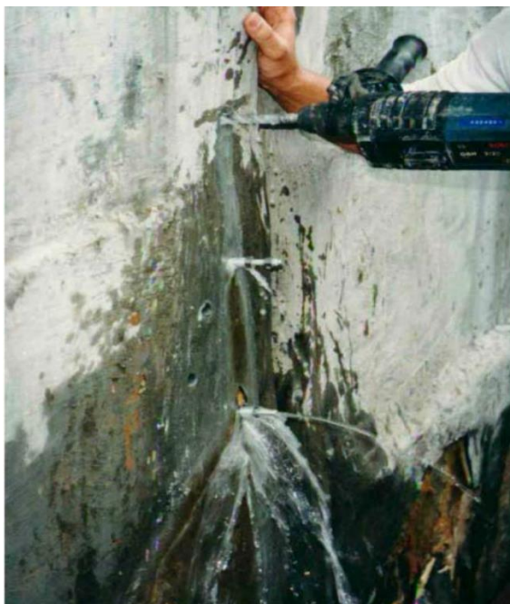
Рисунок 5 – Установка иньекторов
