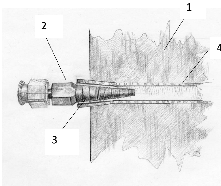
Рисунок 28 – Использование винтового металлического пакера: 1 – бетон; 2 – пакер; 3 – трубка ПВХ; 4 – пробуренное отверстие
