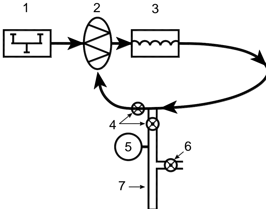
Рисунок 7 – Циркуляционный способ подачи раствора:
