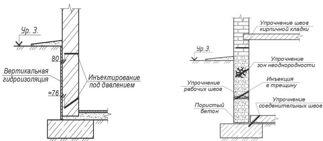
Рисунок 12 – Схемы гидроизоляции
