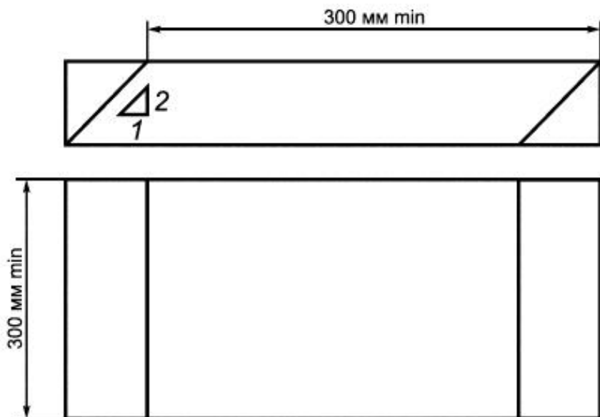
Рисунок И.4 - Размеры верхней части сдвижного короба
