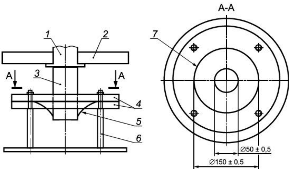
Рисунок Е.2 - Пример зажимного приспособления
