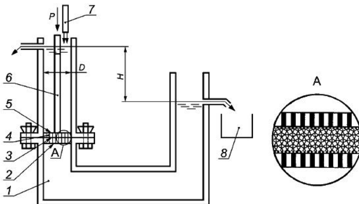
Рисунок Д.1 - Пример схемы прибора для определения водопроницаемости геосинтетических материалов
