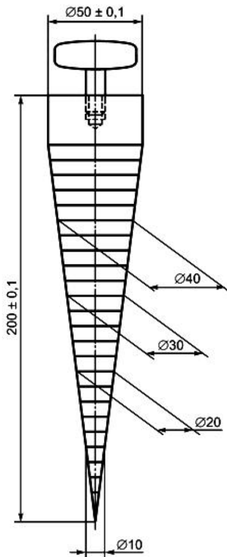
Рисунок Л.5 - Пример измерительного конуса
